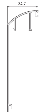
P-1004 0,770 kg/m
