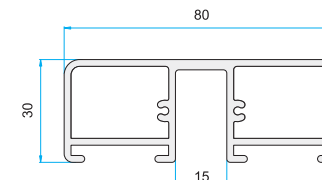
P-AL7116 1,60 Kg/m
