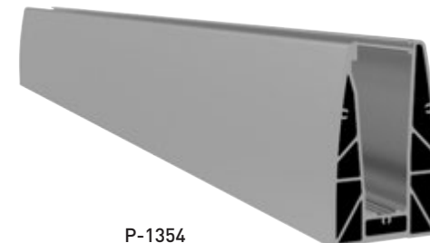
P-1354 4,50 Kg/m
