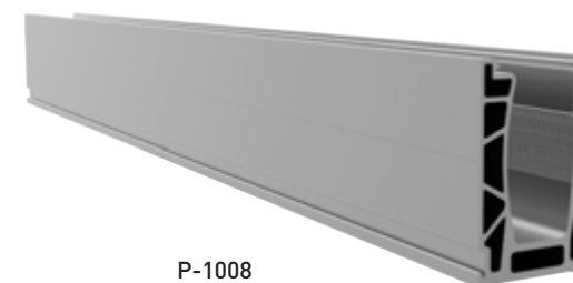
P-1008 5,852 kg/m
